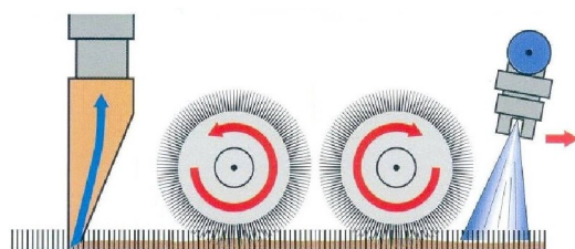
Sistema ad iniezione-estrazione con spazzole contro-rotanti
